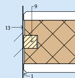
2.12.3 Wandaansluiting
