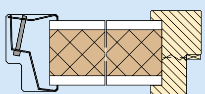
2.12.5 Kozijnaansluiting
