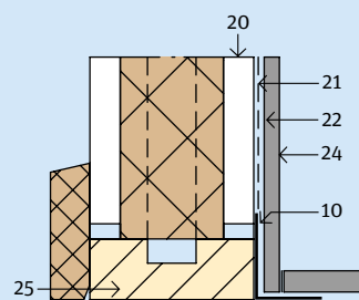
2.11.8 Vloeraansluiting natte cel
