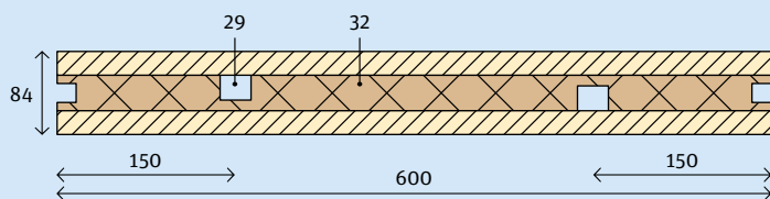
2.15.1 Opbouwelement
