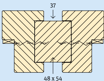
2.11.1 Tussenstijl
