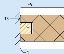
2.10.3 Wandaansluiting
