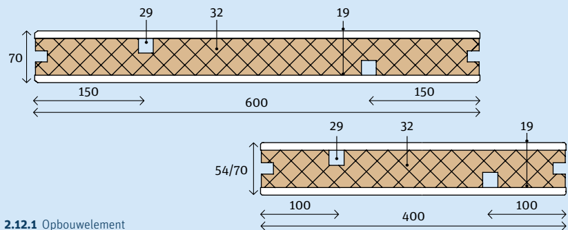
2.12.1 Opbouwelement
