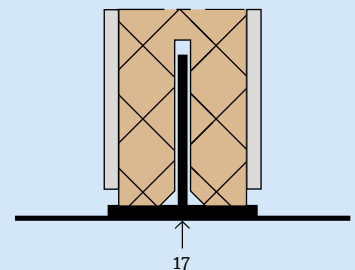
2.14.7 Vloeraansluiting
