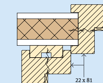
2.10.6 Kozijnaansluiting
