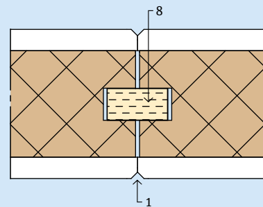
2.12.2 Koppeling
