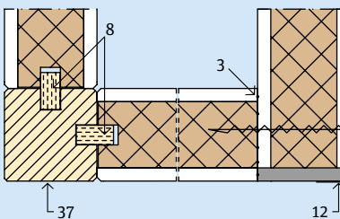
2.12.4 Hoekverbinding
