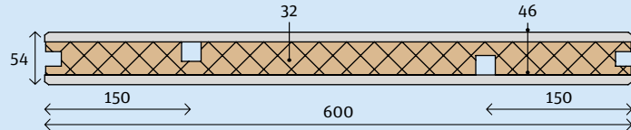
2.14.1 Opbouw wandelement
