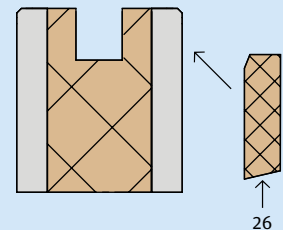
2.14.5 Bovendetail
