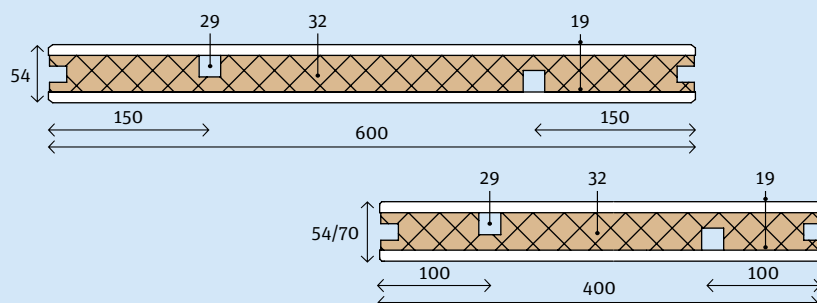
2.10.1 Opbouw wandelement
