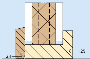
2.11.6 Vloeraansluiting
