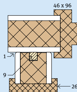
2.12.6 Ontmoeting / kozijnaansluiting / beëindiging
