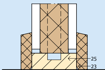
2.11.7 Vloeraansluiting
