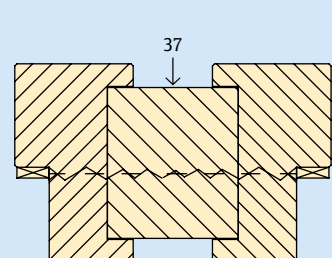
2.12.7 Tussenstijl
